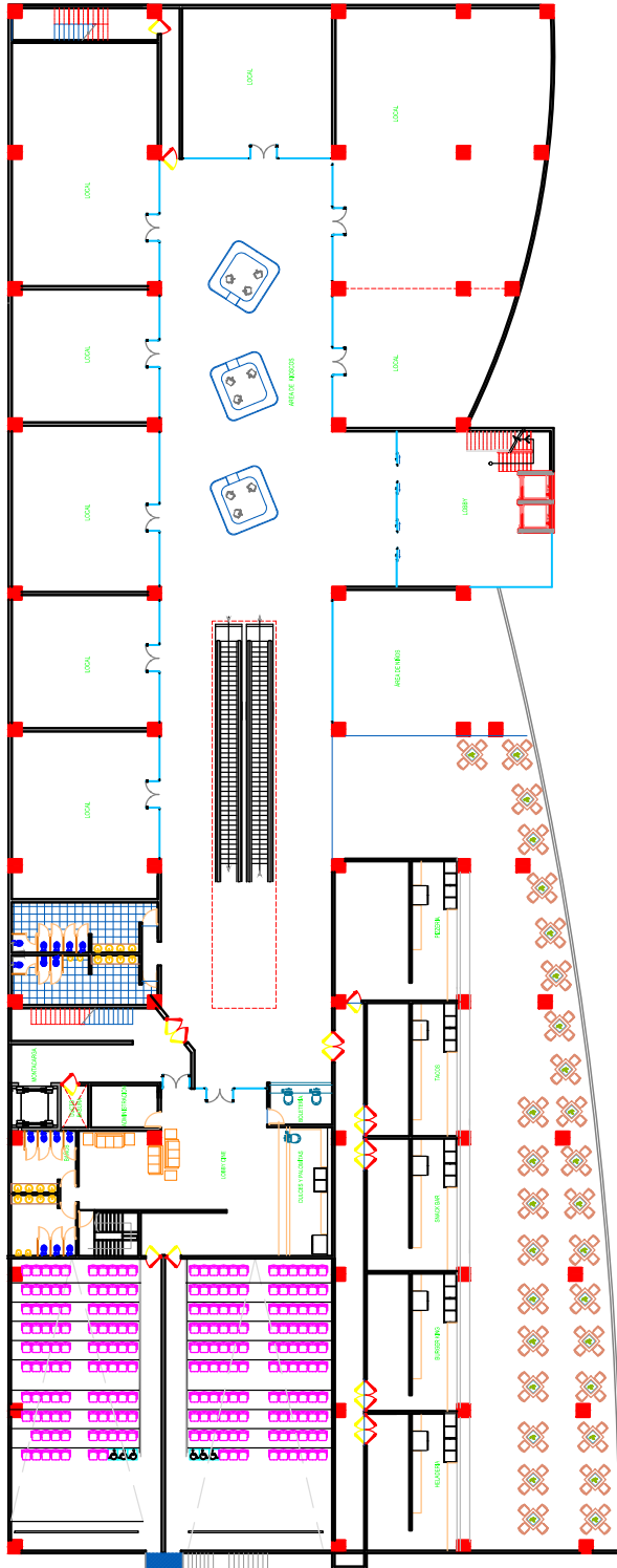
PLANTA ARQUITECTÓNICA PLAZA COMERCIAL 2DO NIVEL ESC. 1/50
